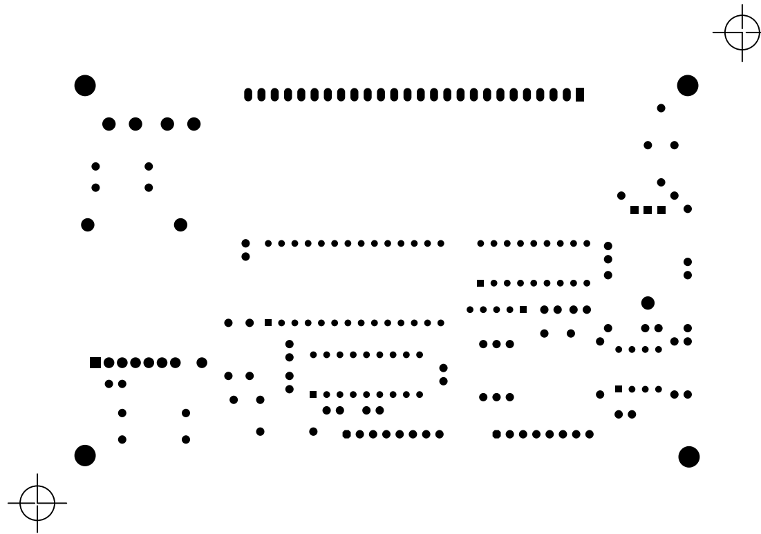
VFD 11 Digit Display Rev EC
